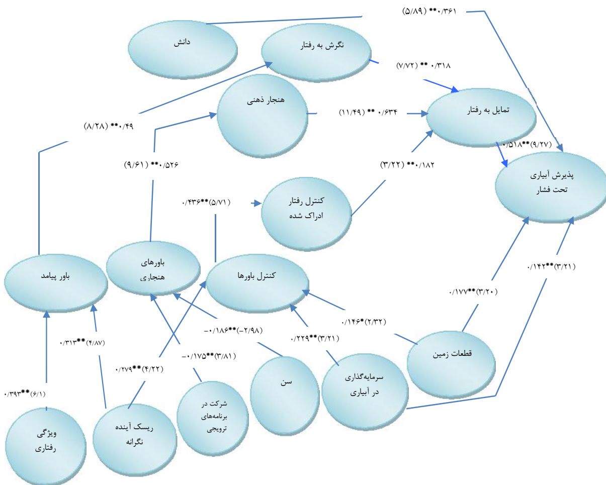
نگاره ۲- نمودار نهایی تحلیل مسیر
